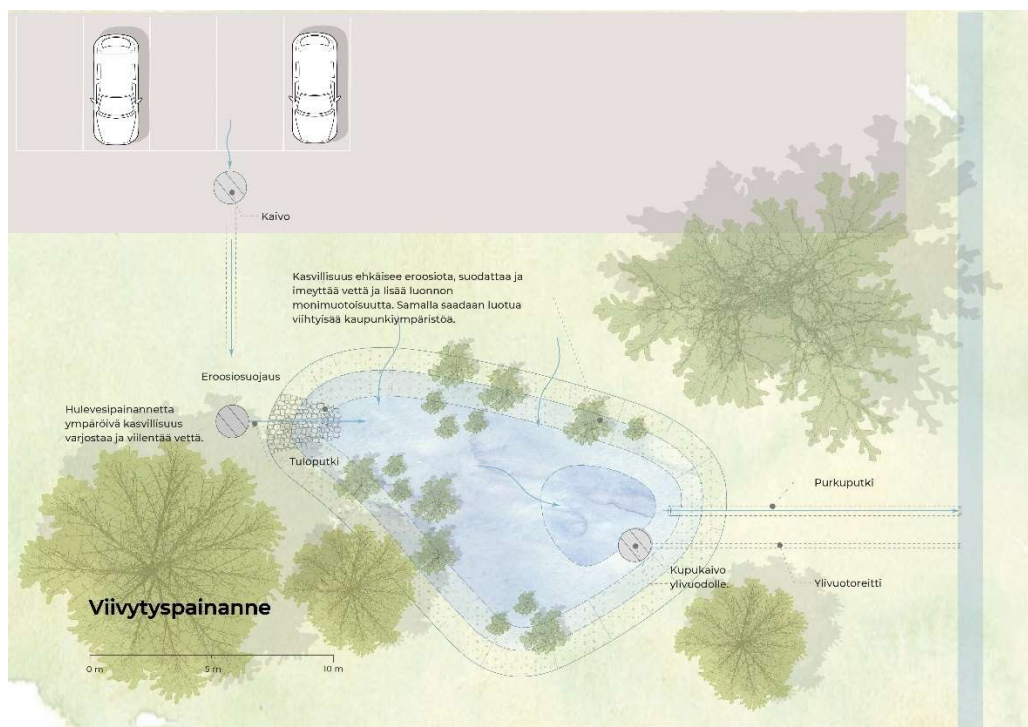
Kuva 10. Viivytyspainanteen tyypik kuva © Destia Oy.
