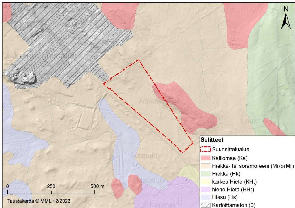
Kuva 4. Suunnittelualan maaperä. Pohjamaalajit © GTK 2023.
