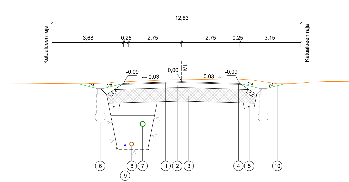
TYYPPIPOIKKILEIKKAUS - PLV 0-46.0 ja 189.4-196.4 (PL 30)
