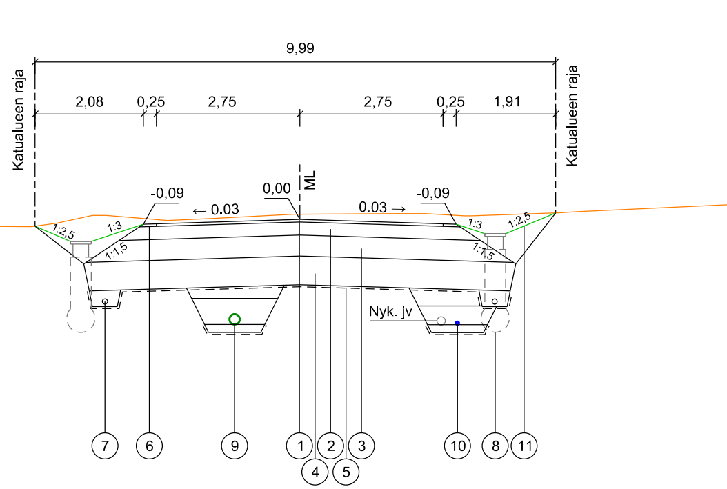
TYYPPIPOIKKILEIKKAUS - PLV 46.0-189.4 ja 196.4-385.6 (PL 230)
